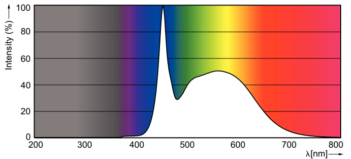
LEDtube HF 1500mm SO 25 W /865 T8
